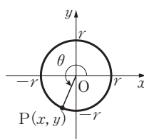
三角関数の値の符号
